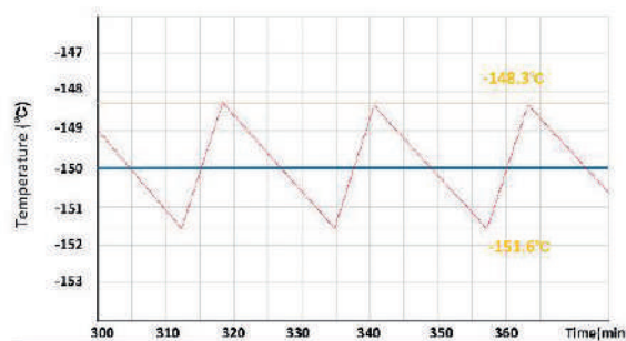
Flutuação da temperatura interna em ambiente a 25°C, sem carga
